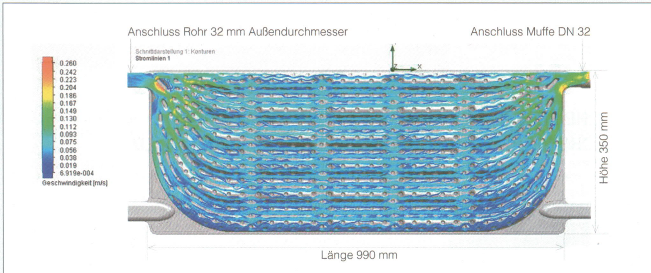
Bild 3: Das besondere Design der GeoCollect-Absorber aus robustem Polypropylen ermöglicht hohe Entzugsleistungen auf kleiner Fläche.
